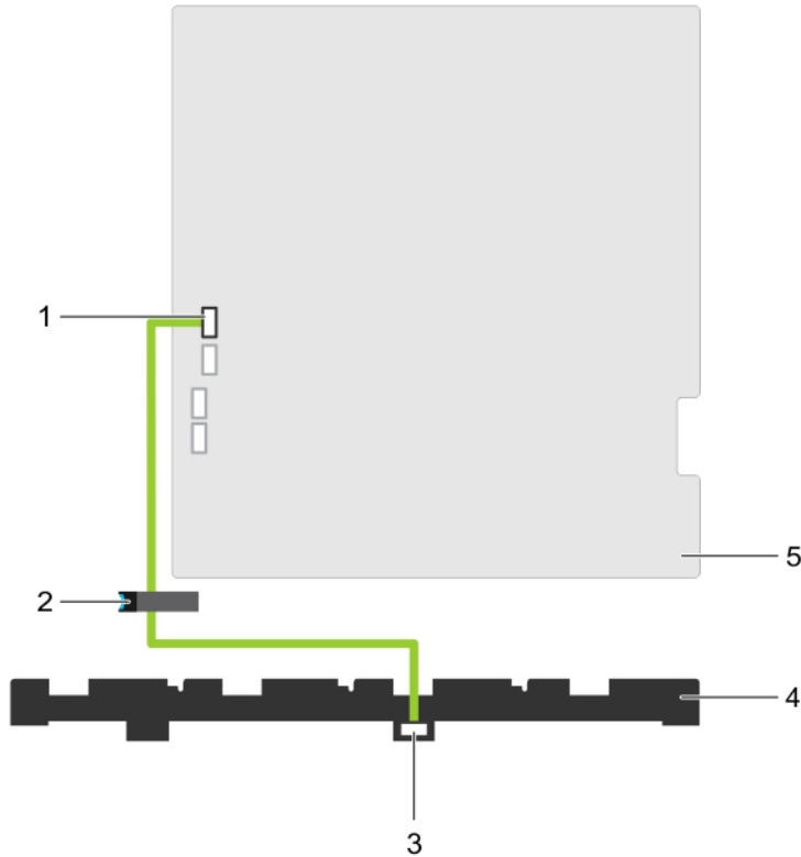
그림 27. 케이블 연결 다이어그램 – 3.5인치 (x4) SAS/SATA 후면판
