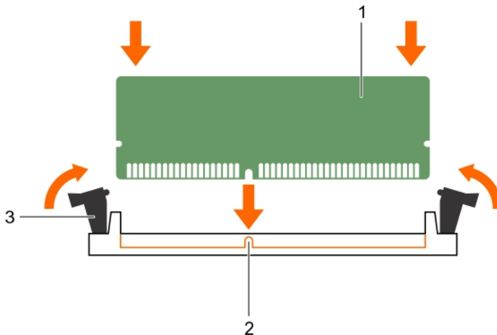
그림 13. 메모리 모듈 설치
