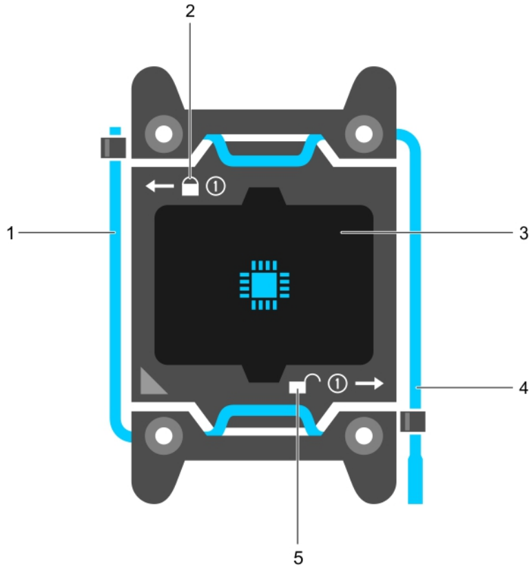
그림 21. 프로세서 실드 레버 열기 및 닫기 시퀀스
