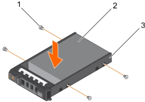
그림 18. 핫 스왑 가능한 하드 드라이브 캐리어에 핫 스왑 가능 하드 드라이브 설치
