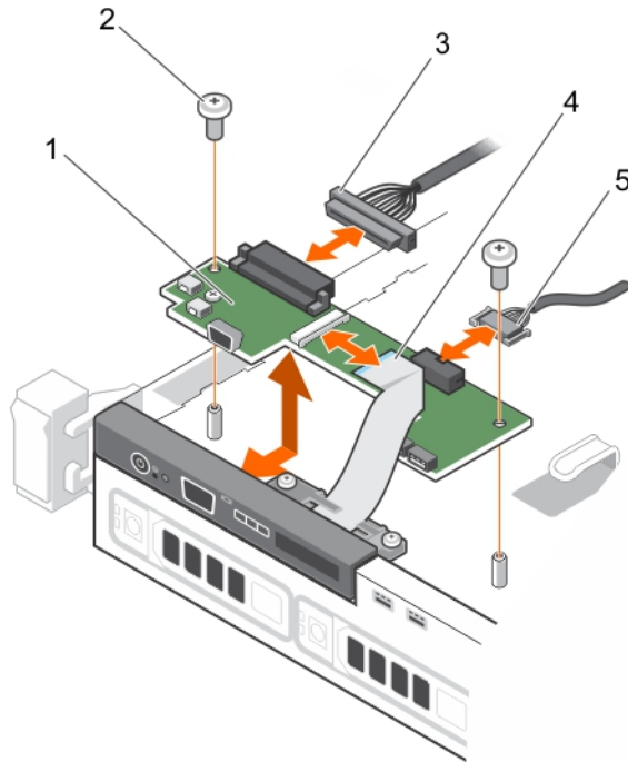
그림 29. 제어판 모듈 분리 및 설치 - 4개의 하드 드라이브 새시
