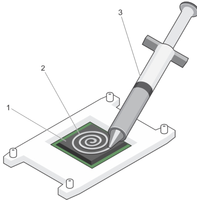
그림 23. 프로세서 상단에 열 그리스를 적용
