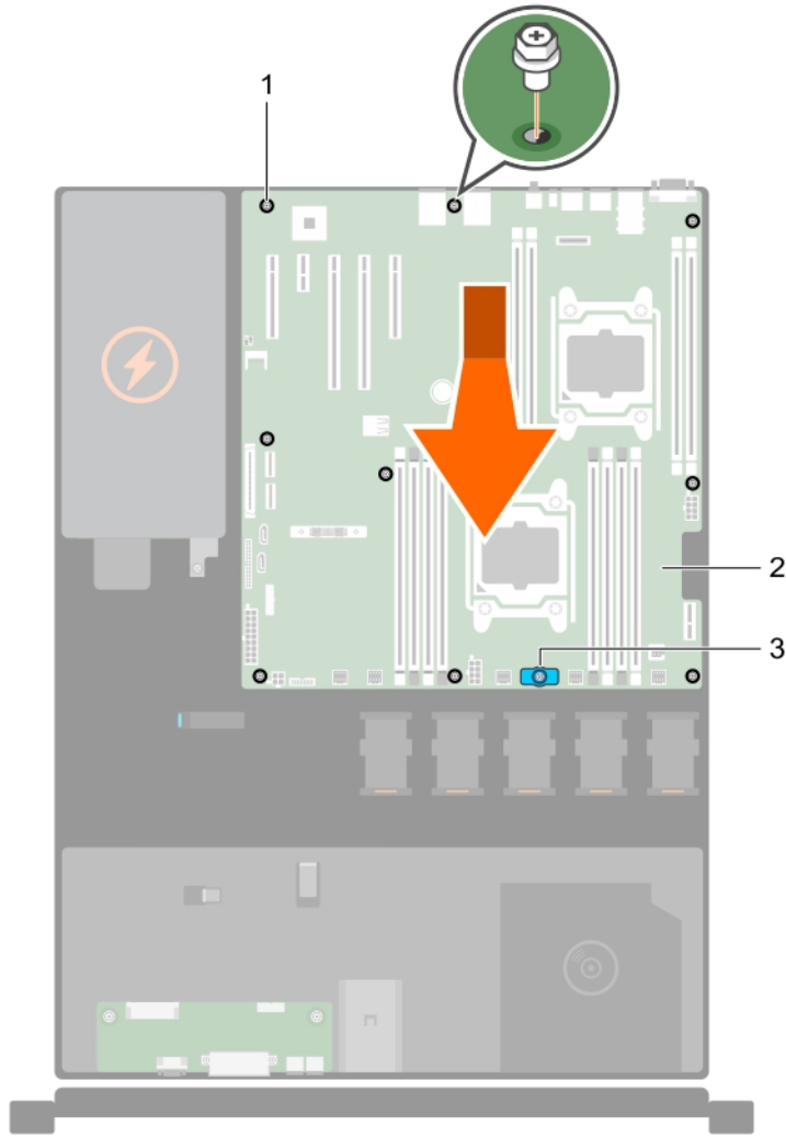
그림 31. 시스템 보드 분리 및 설치
