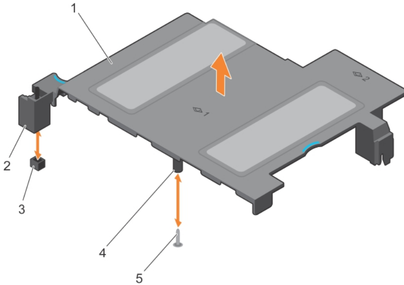
그림 10. 냉각 덮개 분리 및 장착
