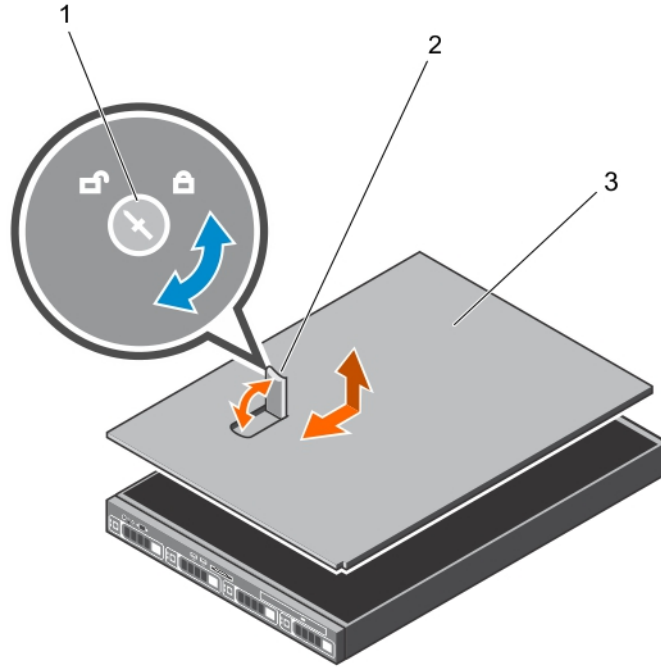
그림 8. 시스템 덮개 분리 및 설치
