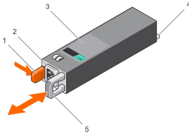
그림 24 . 중복 PSU 분리 및 설치
