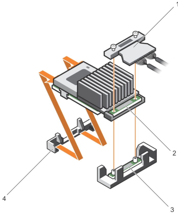
그림 20. 내장형 스토리지 컨트롤러 카드 분리 및 설치
