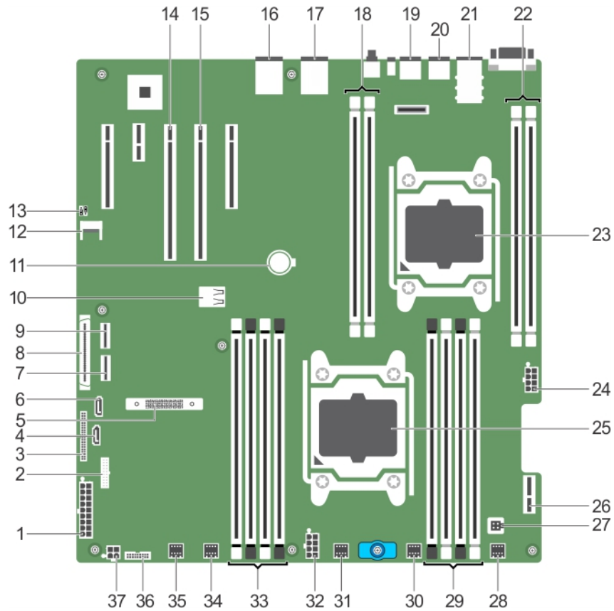
그림 33. 시스템 보드 점퍼 및 커넥터
