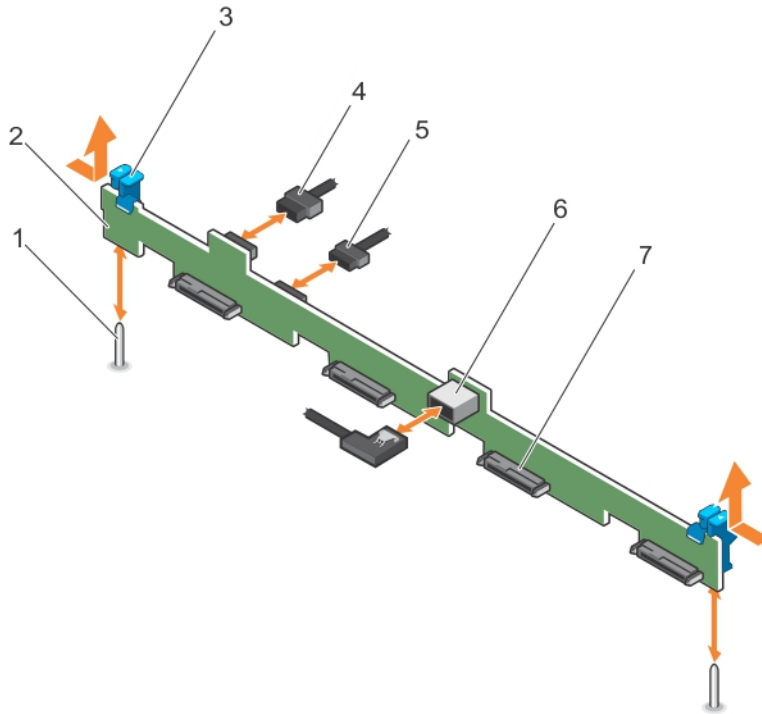
그림 26 . 3.5인치 (x4) SAS/SATA 후면판 분리 및 설치
