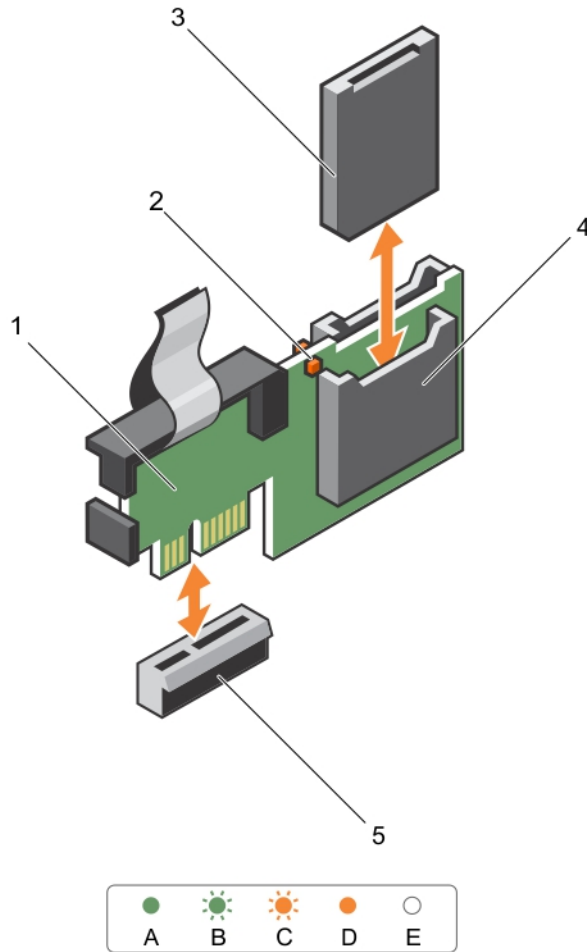
그림 19. 내부 이중 SD 모듈(IDSDM) 분리 및 설치
