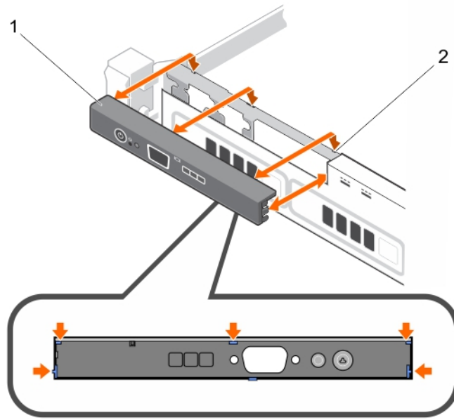
그림 28 . 제어판 분리 및 설치 - 4개의 3.5인치 하드 드라이브 새시
