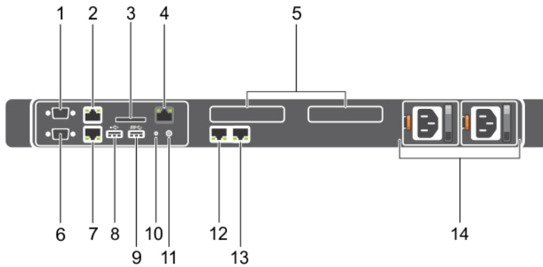
그림 5. 후면 패널 구조 및 표시등
