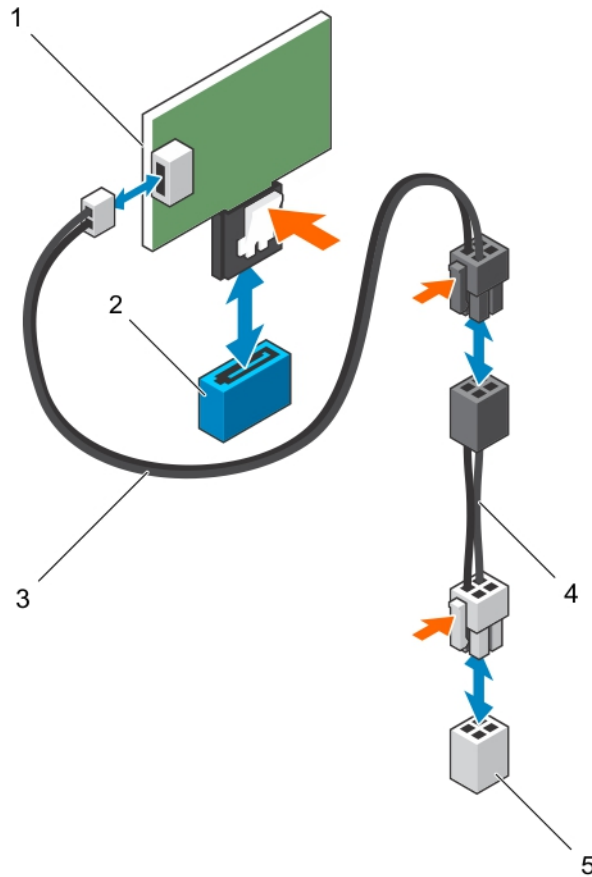
그림 14. SATADOM 분리 및 설치
