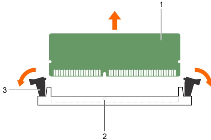
그림 12. 메모리 모듈 분리
