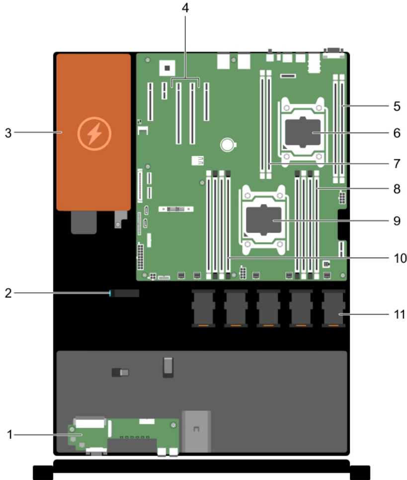
그림 9. 시스템 내부 - 비중복 전원 공급 장치 포함
